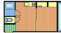
Cタイプ (25.00㎡) DK6.0×和6.0
