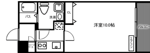
Dtype 04号室
