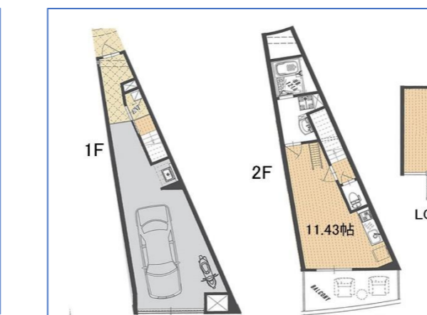
B2タイプ (66.90㎡) LDK11.43×洋5.00×ガレージ
