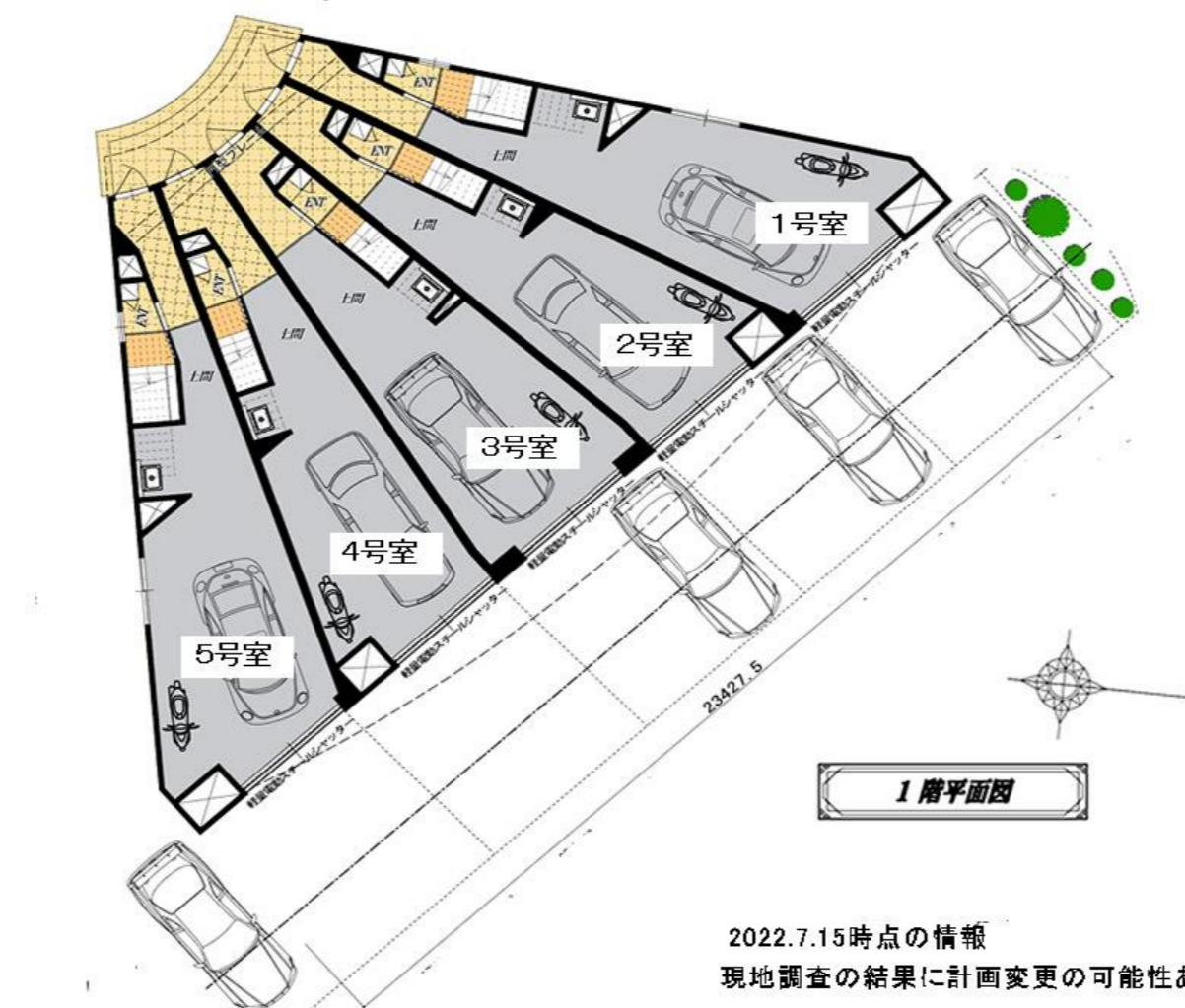
A2タイプ (81.56㎡) LDK11.36×洋4.53×ガレージ
