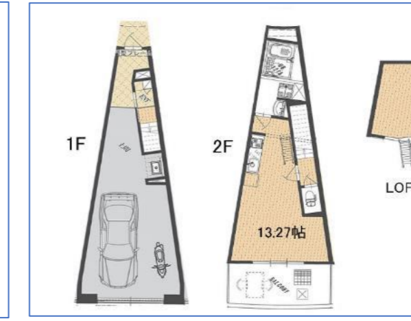
Cタイプ (72.00㎡) LDK13.27×洋5.00×ガレージ
