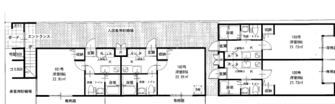
1階 平面図
